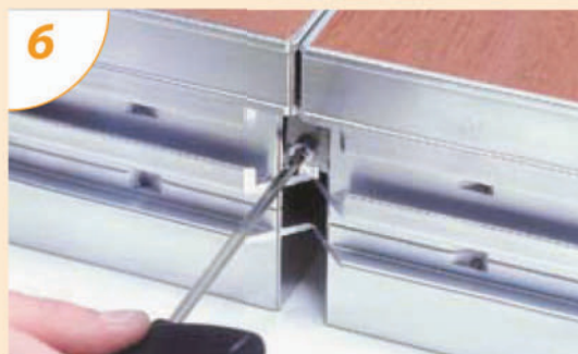
6 Schnellverbinder-kurz , damit sichern Sie die Bühnenelemente untereinander im Randbereich
